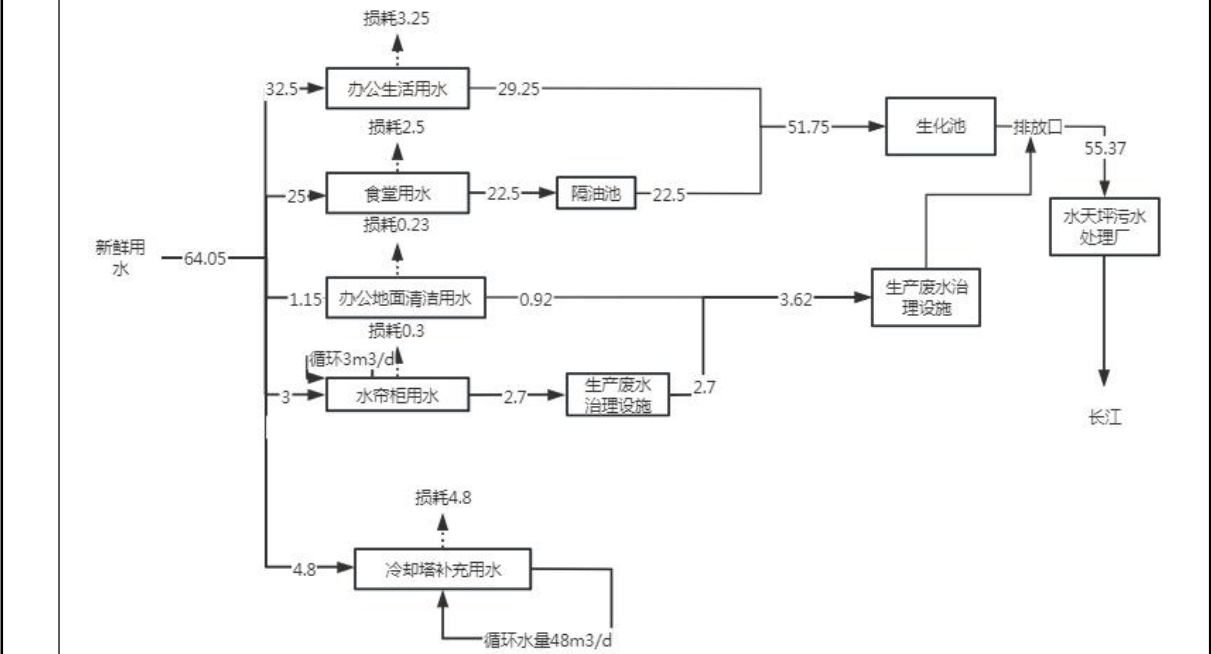
图 2.8-1 改扩建项目水平衡图 (m³/d)
