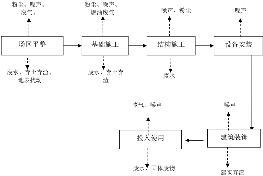
图 2.9-1 拟建项目施工期工艺流程及产污环节图
