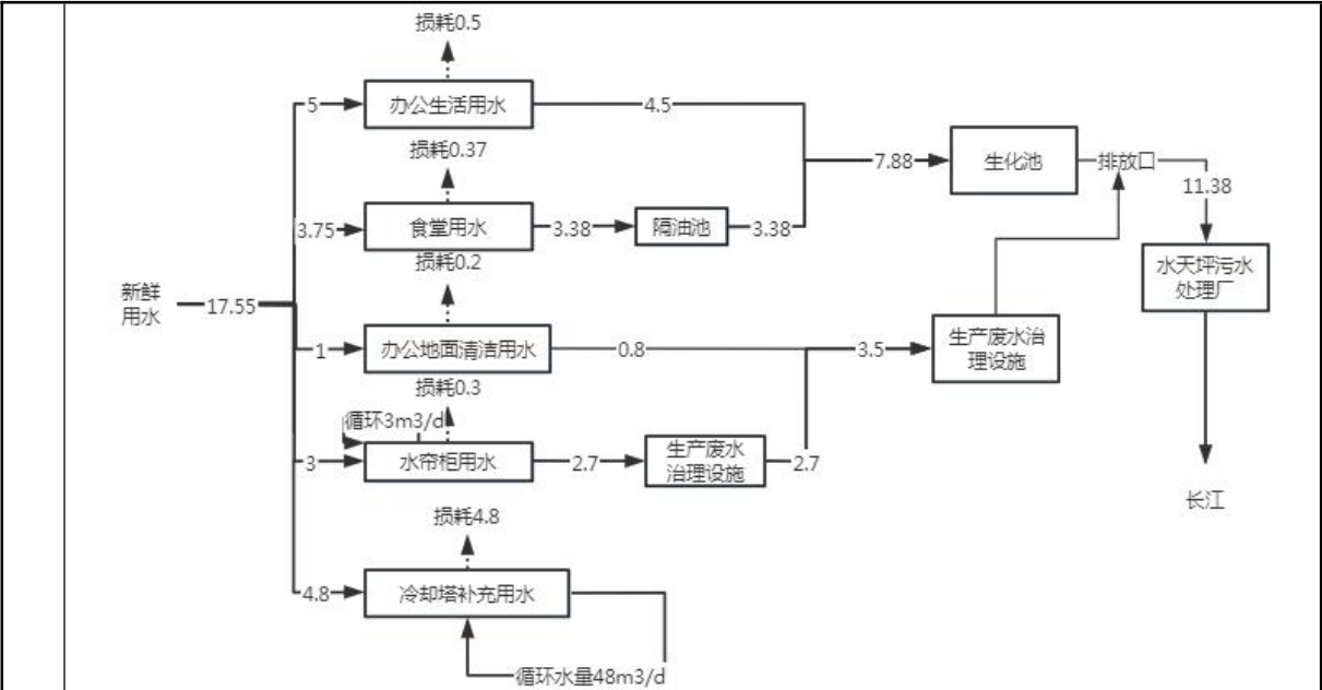
图 2.8-1 改扩建项目水平衡图 (m³/d)
