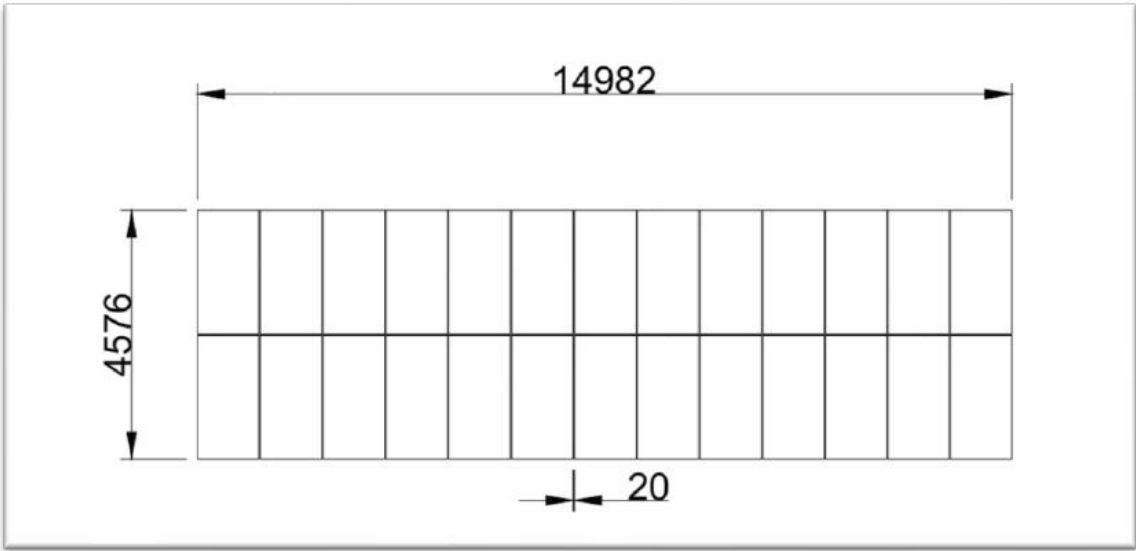
图 2.2-3 组件纵向排列示意图
