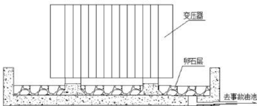
图 5.3-2 事故油坑示意图
