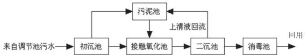
图 5.3-1 生活污水处理工艺流程图
