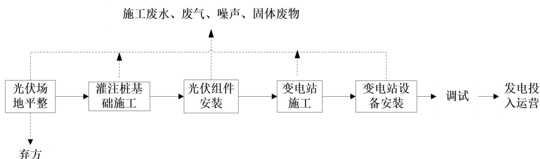
图 2.4-1 本项目施工工艺图
