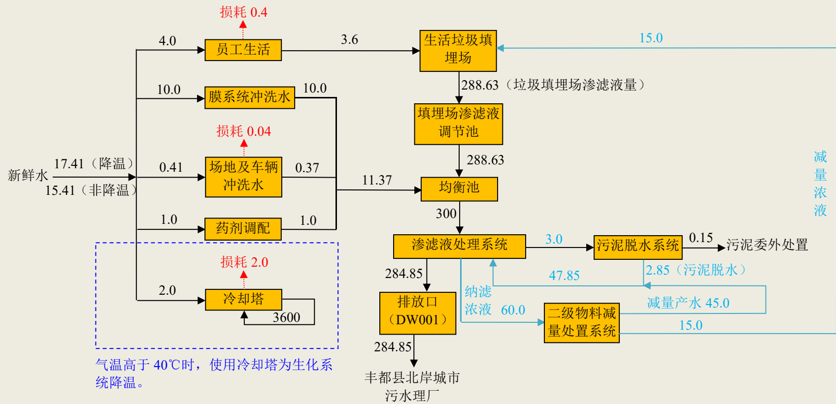
图 2-1 项目水平衡图 (m³/d)
