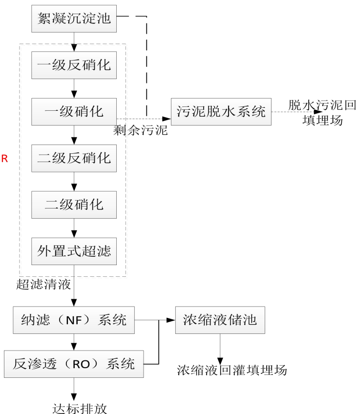
图 2-9 现有工艺流程图
