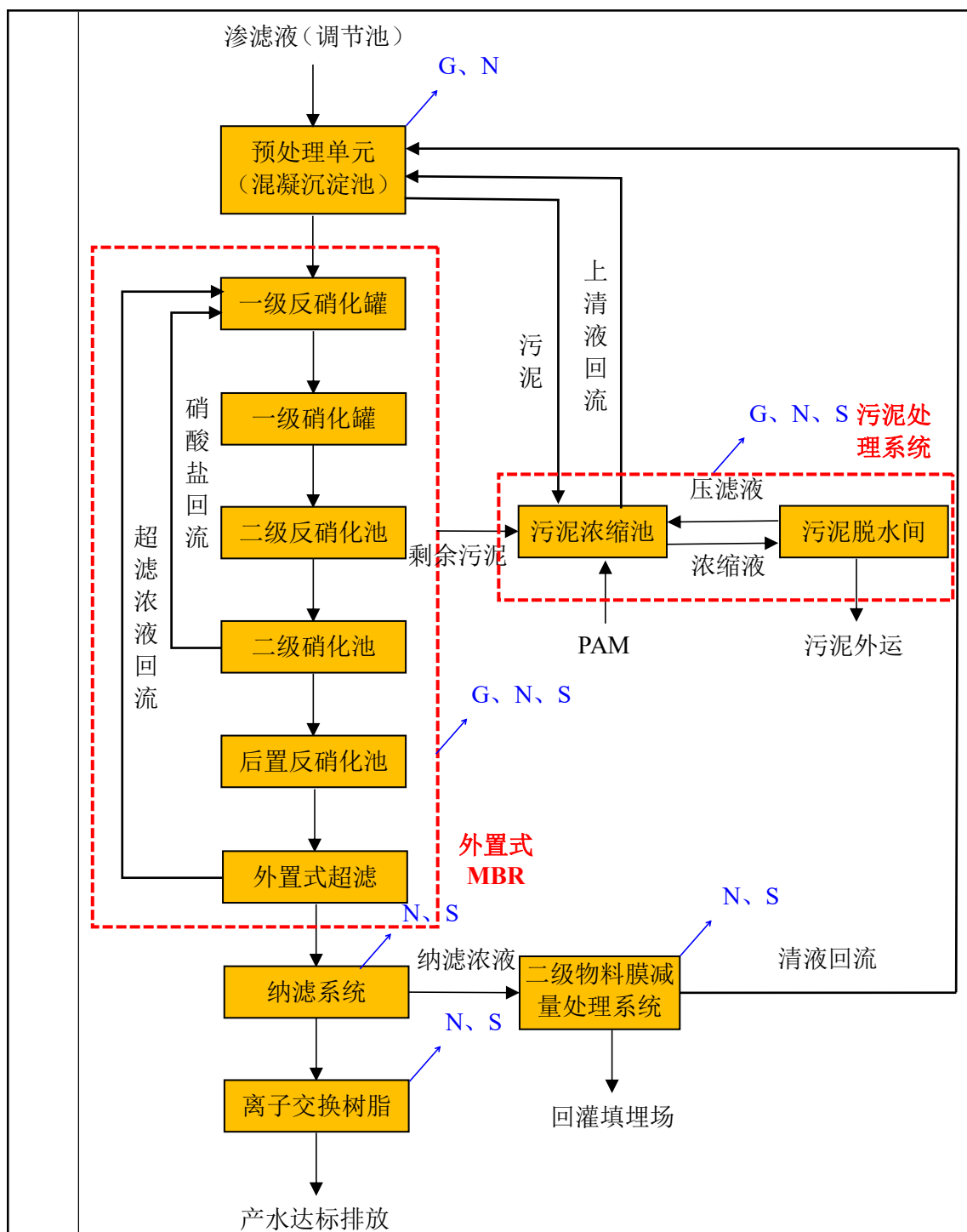
图 2-4 施工期渗滤液应急处理工艺流程及产排污环节
