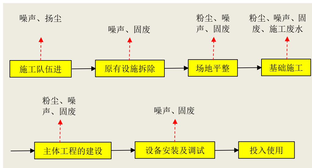
图 2-2 项目施工期施工工艺流程及产污环节
