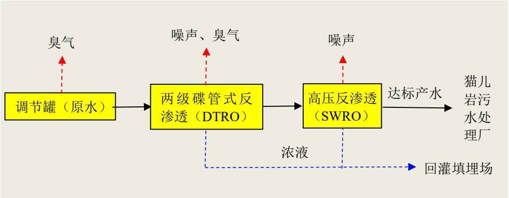
图 2-3 渗滤液应急处理工艺流程及产排污环节
