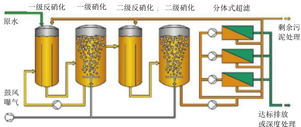
图 2-5 外置式膜生化反应器（MBR）工艺原理图
