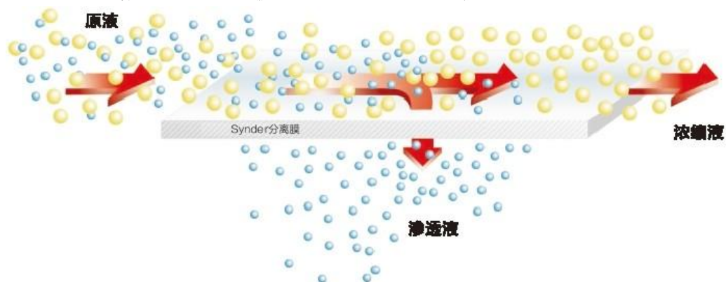
图 2-9 两级物料膜系统原理图
