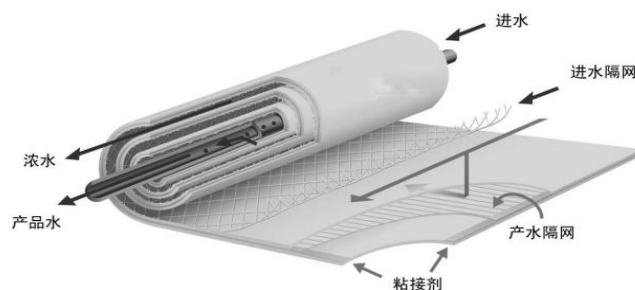
图 2-7 卷式纳滤膜结构图
