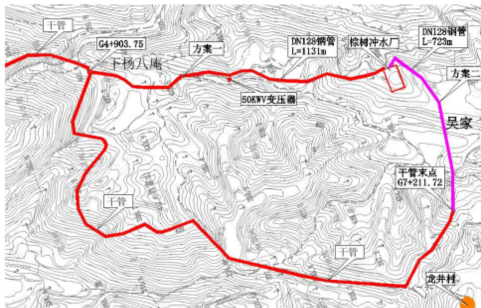
图 1.9-4 棕树冲水厂支管方案比选图
