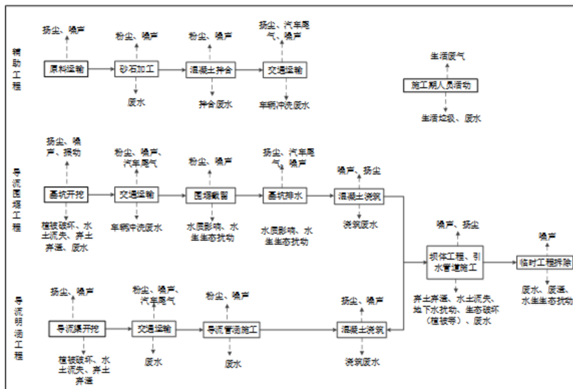
图 3.1-1 水库枢纽工程施工工艺流程及产污环节示意图
