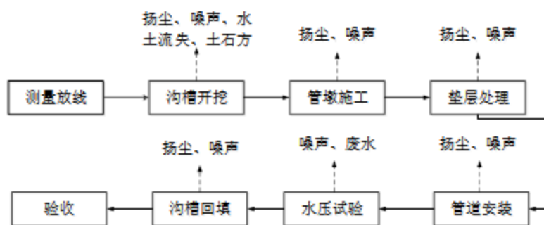
图 3.1-3 输水工程施工工艺流程及产污环节示意图
