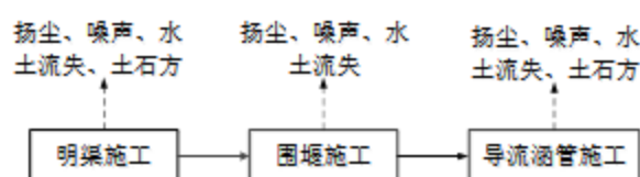
图 3.1-4 导流工程施工工艺及产排污环节图
