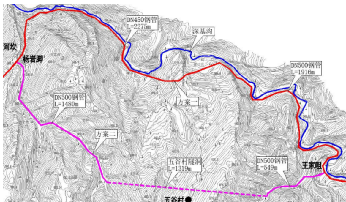
图 1.9-1 项目输水干管选线比选图
