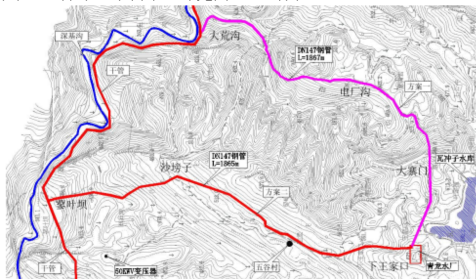
图 1.9-3 青龙水厂支管方案比选图
