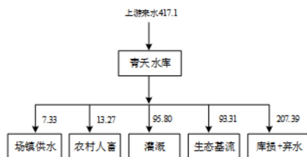
图 2.3-1 青天水库水量平衡图 单位：万 \text{m}^3
