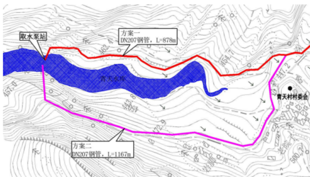
图 1.9-2 青天支管选线方案比选图
