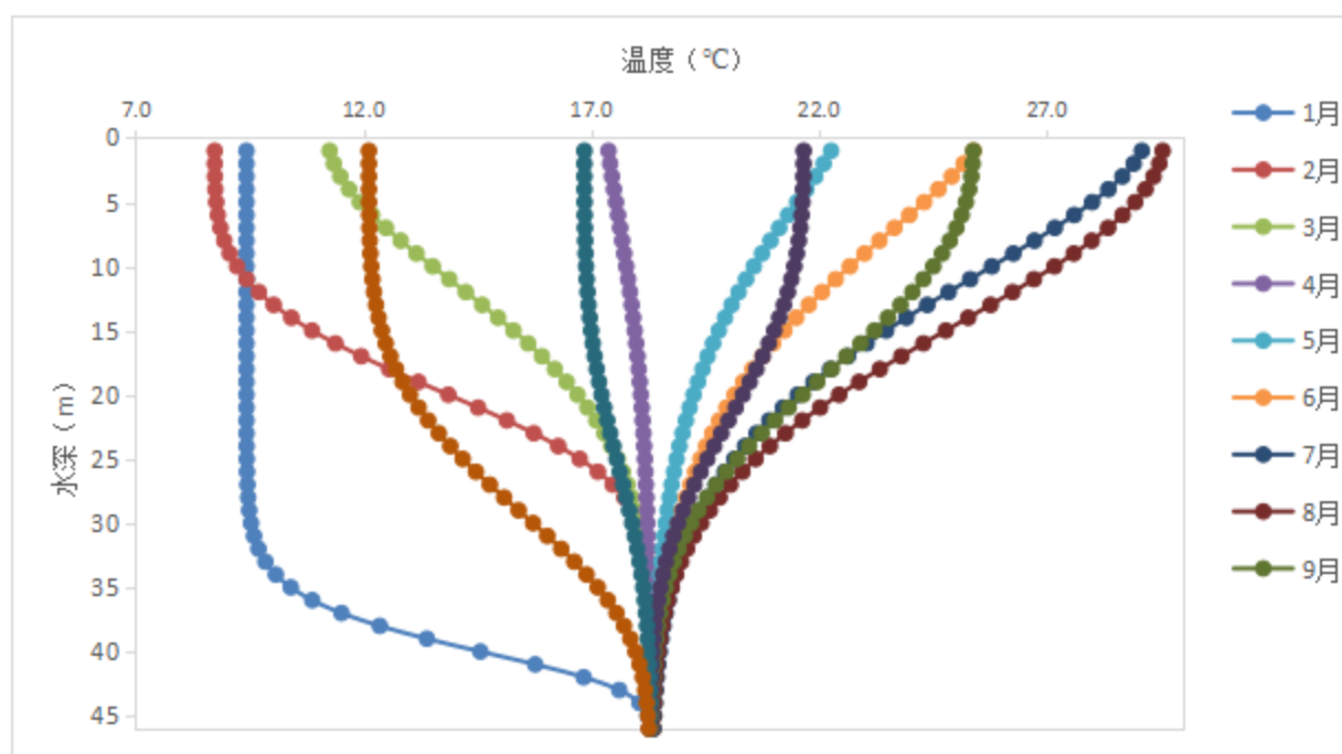
图 5.3-1 青天水库坝前水深垂向分布图
