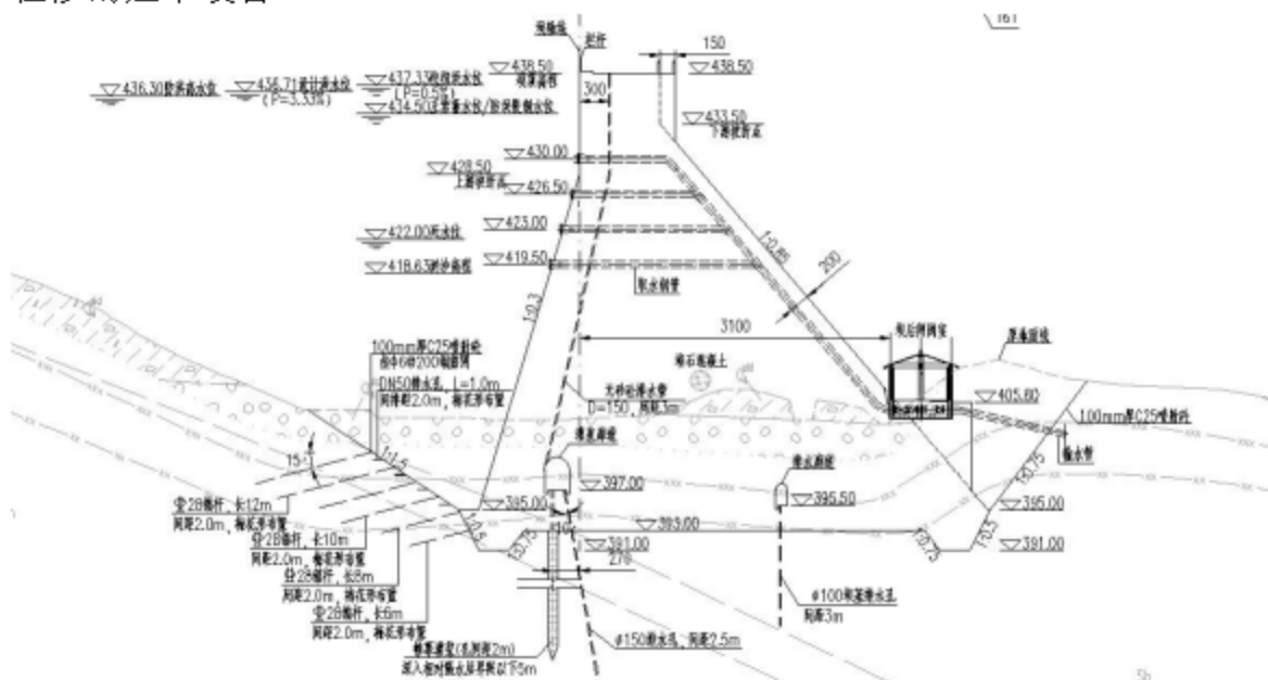
图 2.5-3 坝内取水口布置图
