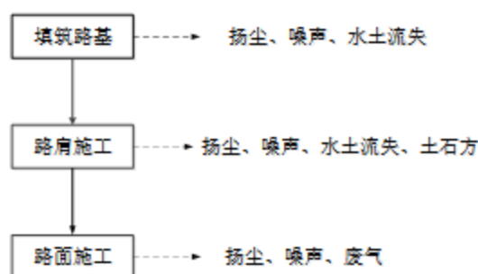
图 3.1-2 道路工程施工工艺流程及产污环节示意图
