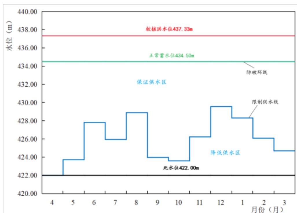
图 2.3-2 水库日常运转方式
